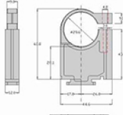
supporto alto per collettore lineare 3/4"
