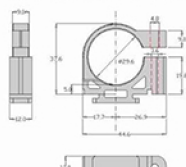
supporto basso per collettore lineare 3/4"
