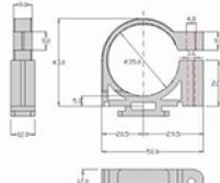
Supporto basso per collettore lineare da 1"
