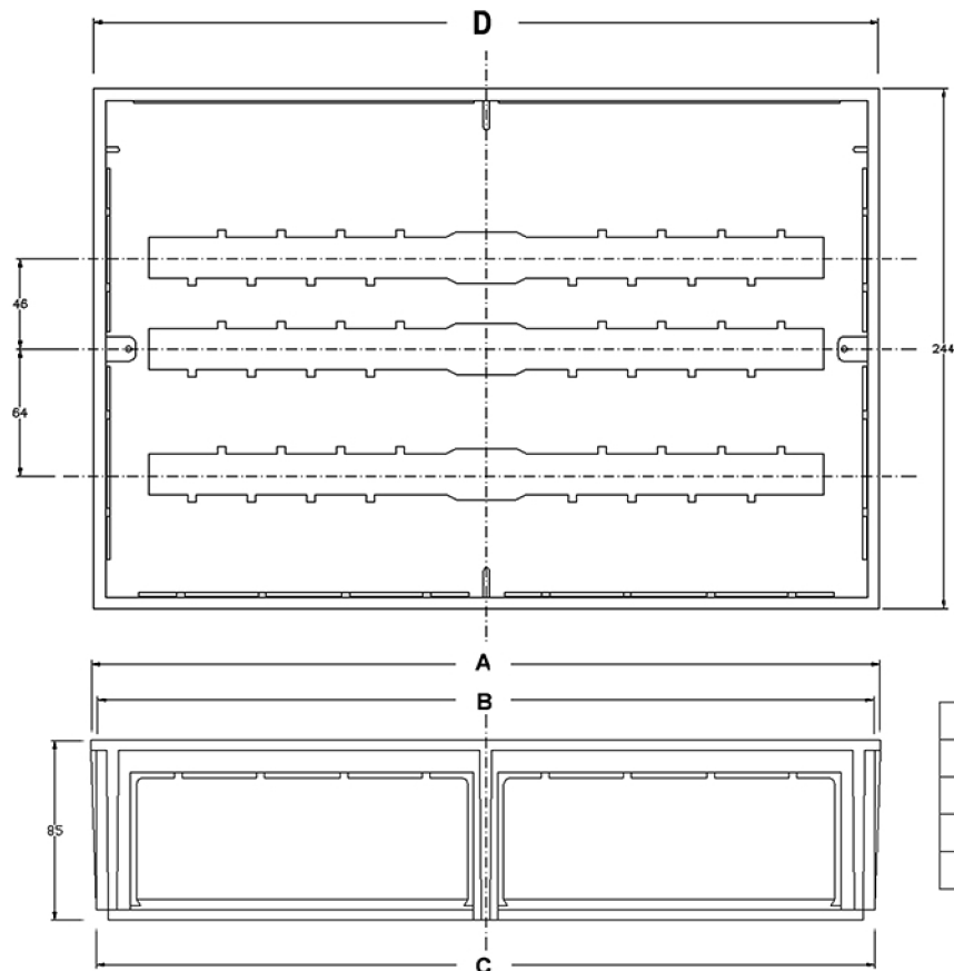
supporto basso per collettore lineare 3/4"
