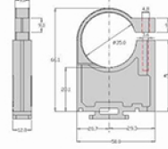
Supporto alto per collettore lineare da 1"
