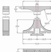
supporto per collettore complanare 3/4" e 1"
