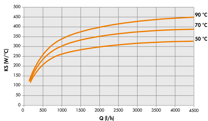
Scambiatore inferiore
