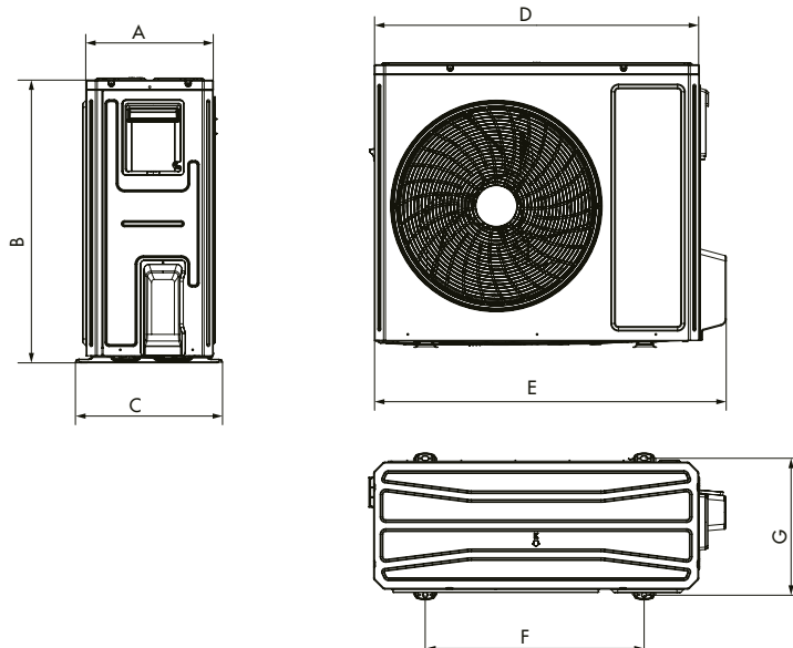
UNITÀ ESTERNA TRIFASE
