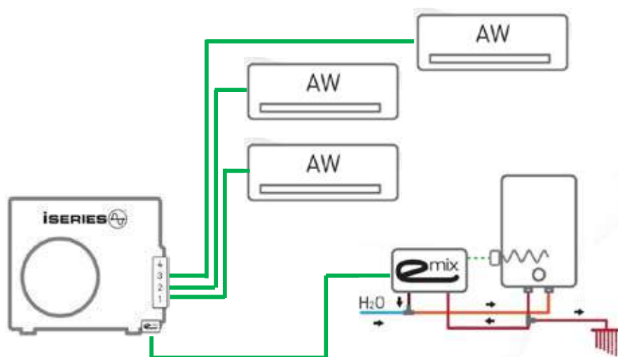
Impianto multisplit per applicazioni residenziali con produzione di ACS
