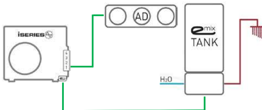
Impianto monosplit con produzione di ACS
