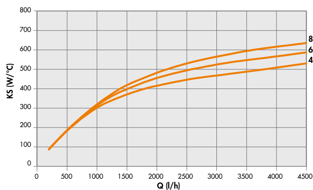
Scambiatore superiore
