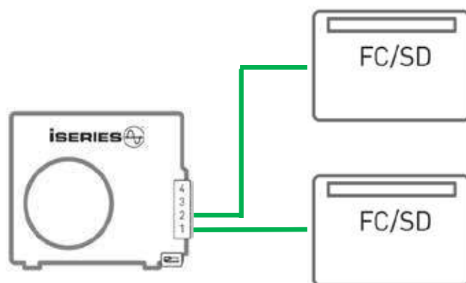
Impianto mono/multisplit per computer room
