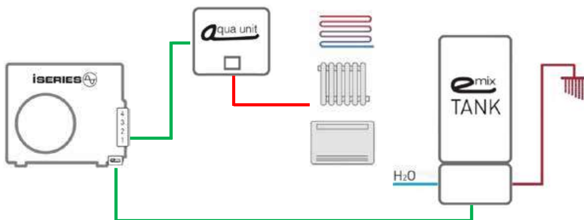
Impianto idronico con produzione di ACS
